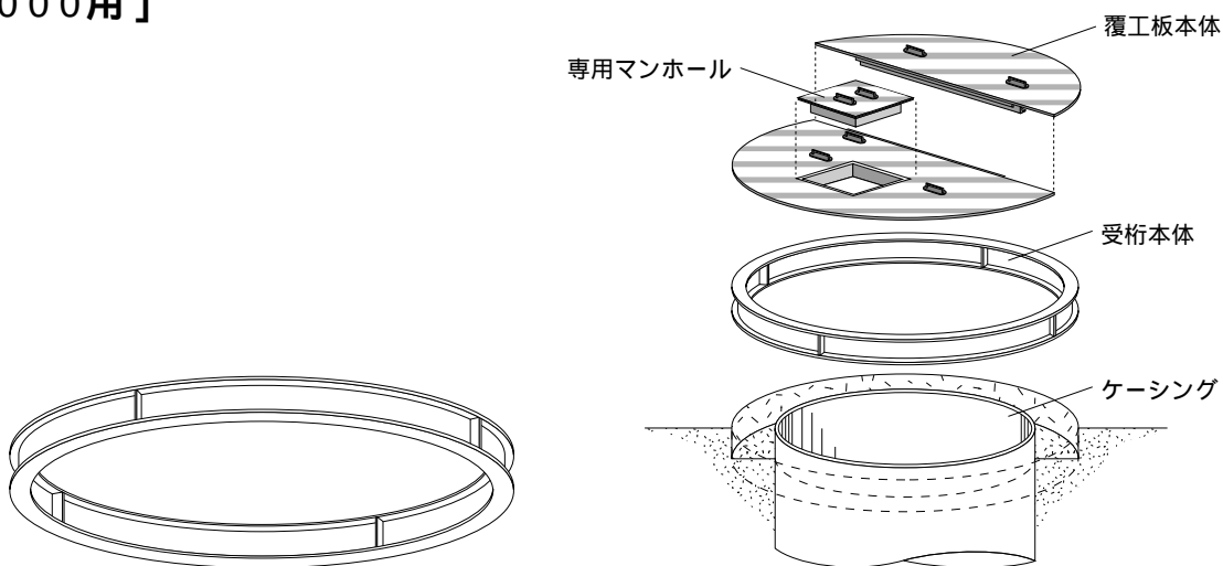
下方斜視図
