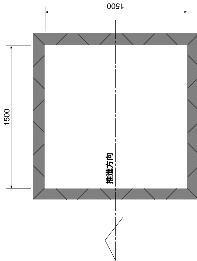
発進坑(矢板)
